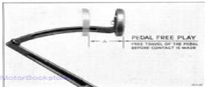
Fig. 67—Brake Pedal Free Play
