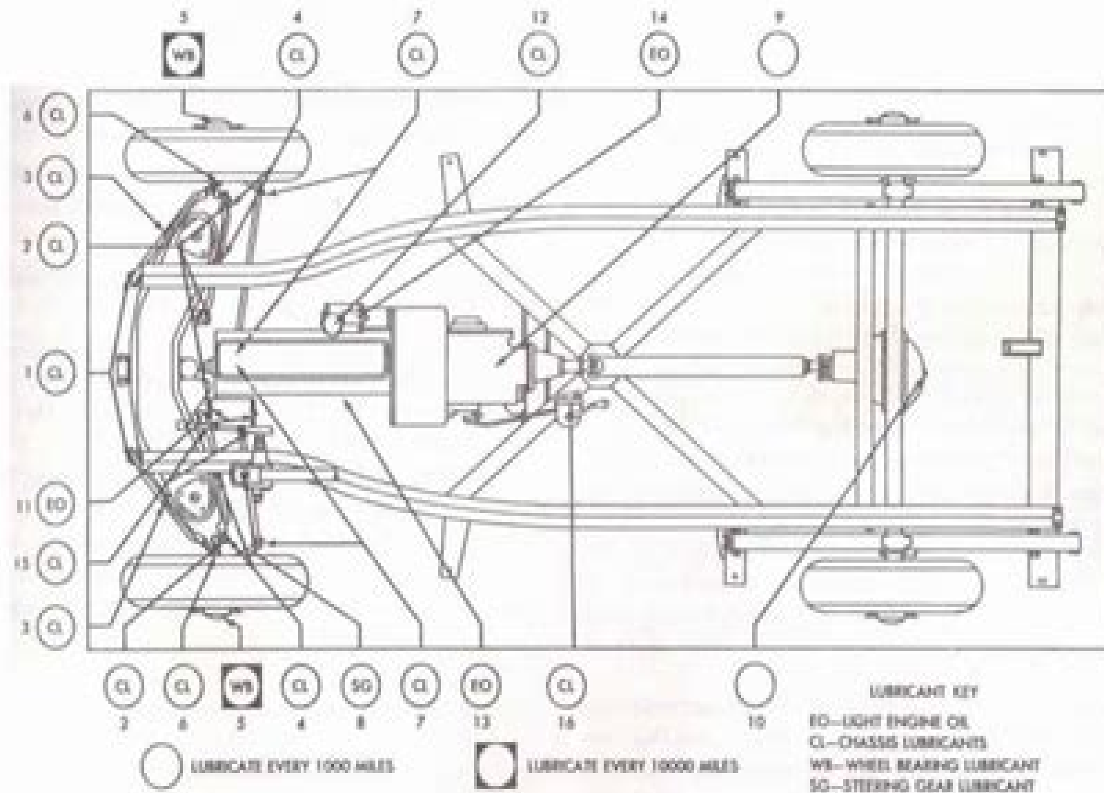
Fig. 40—Lubrication Chart
