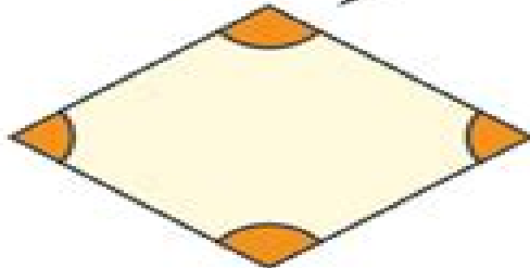
Rhombus
